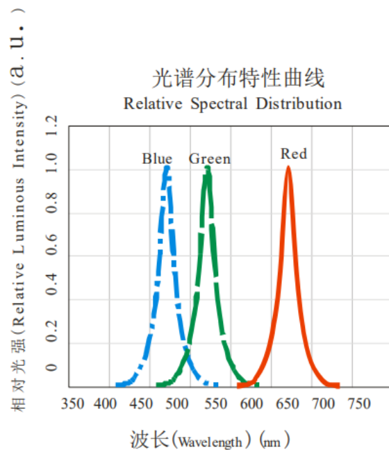
Wavelength(nm)主波长
