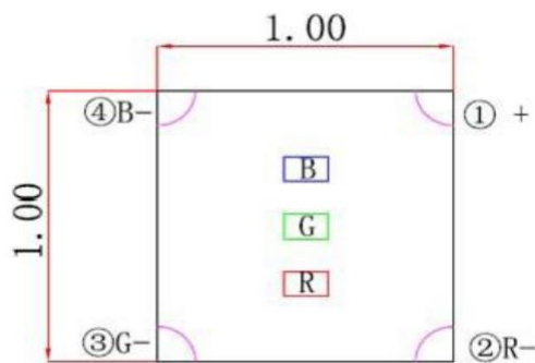
正视图
