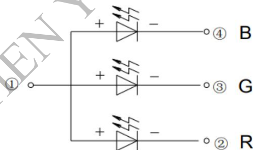
电路图
