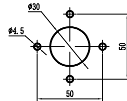
HGL、HGLi-125~630隔离开关柜外手柄安装尺寸
