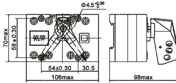
■ HGL、HGLi-80~100 Isolation switch
