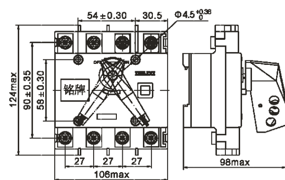
■ HGL、HGLi-80~100 Isolation switch
