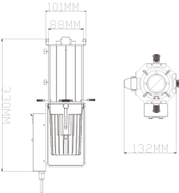
最大光斑 - 30°
