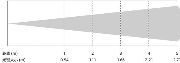
最大光斑 - 30°
