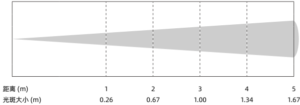
最小光斑 - 15°
