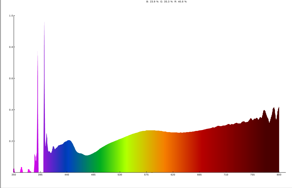
光谱图
