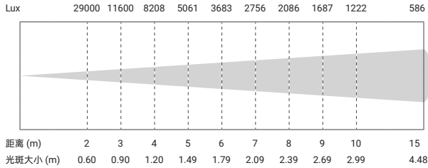
最小光斑 -18°
