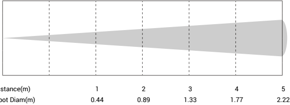
Min. Spot - 25°
