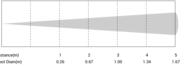
Min. Spot - 15°
