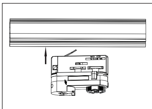
步骤 3 将轨道头装入轨道
