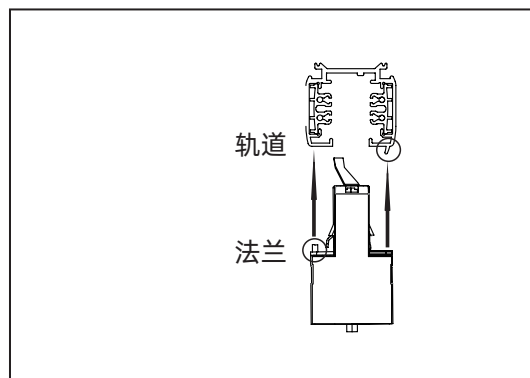
步骤 2 注意轨道头凸起位置和轨道凸起的位置
