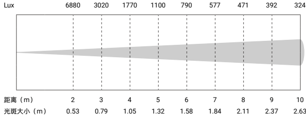
最小光斑 - 15° 5600K
