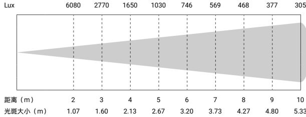
最大光斑 - 30° 5600K
