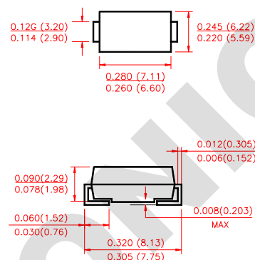
DO-214AB(SMC)
