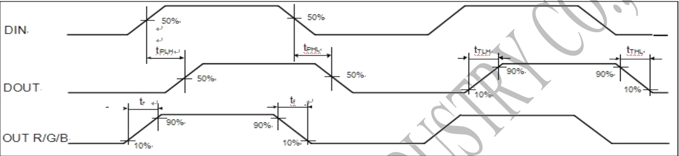
Fig. 动态参数测试示意图
