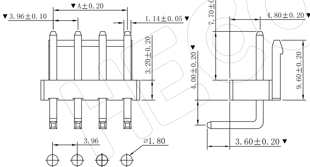
P. C. B. LAYOUT
