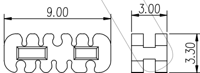
线夹尺寸图
