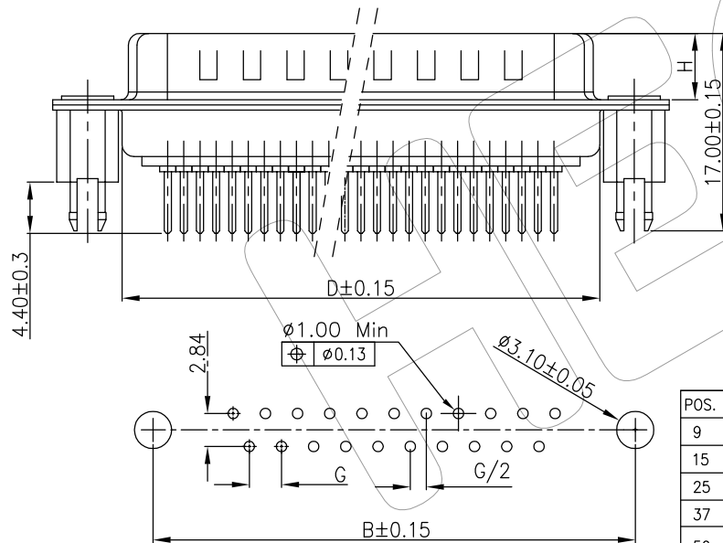
P.C.B LAYOUT
