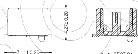
A-A SECTION
