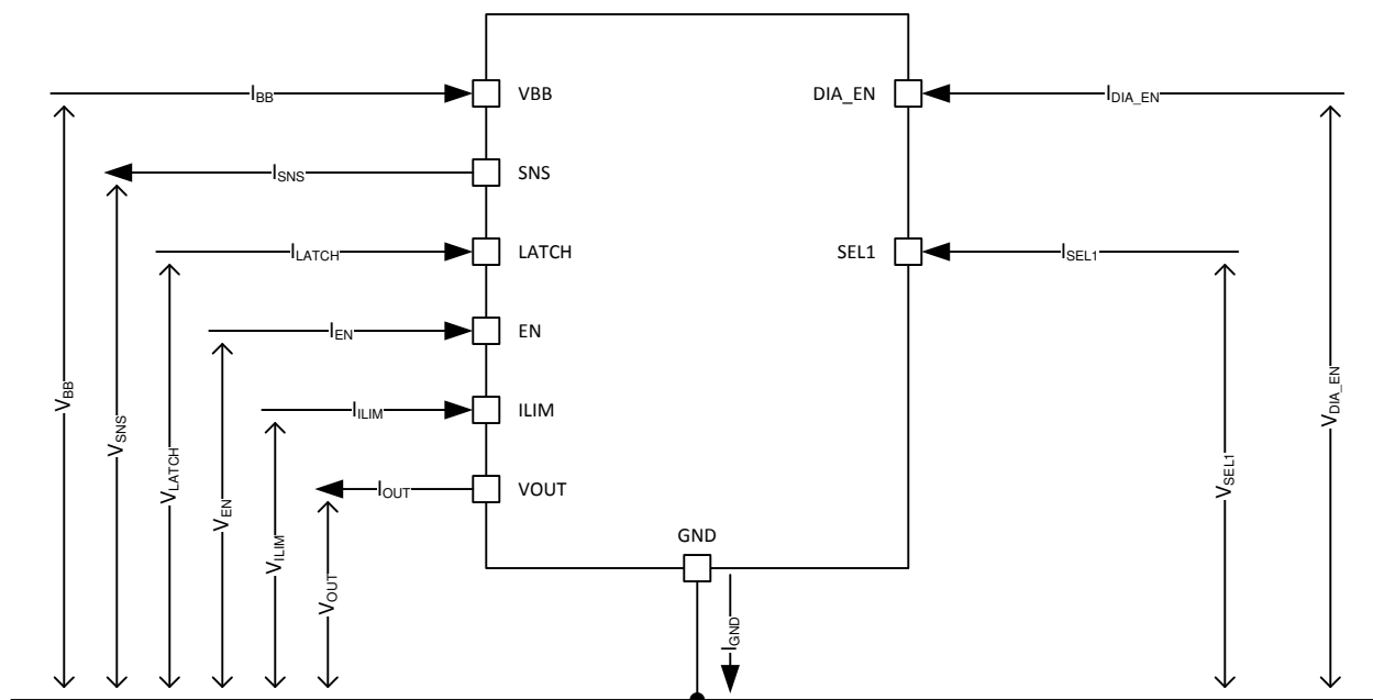
Figure 29. Parameter Definitions
