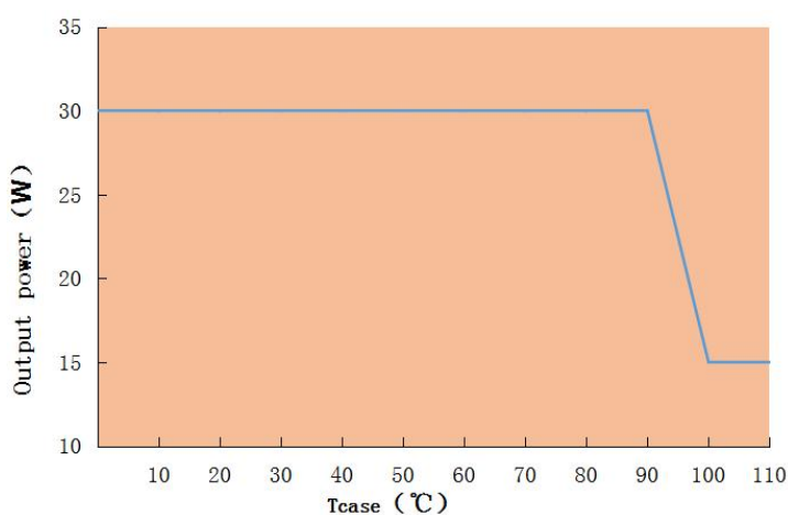
Output power VS Tcase(HVC-30W-56A/B)
