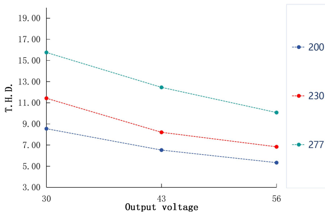
T.H.D. VS Output voltage
