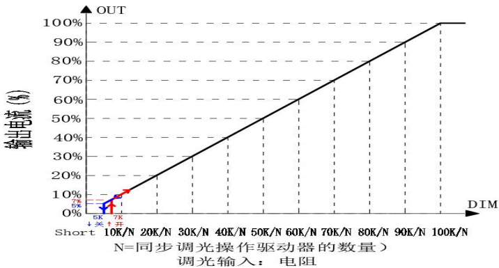
电阻调光（100K）
