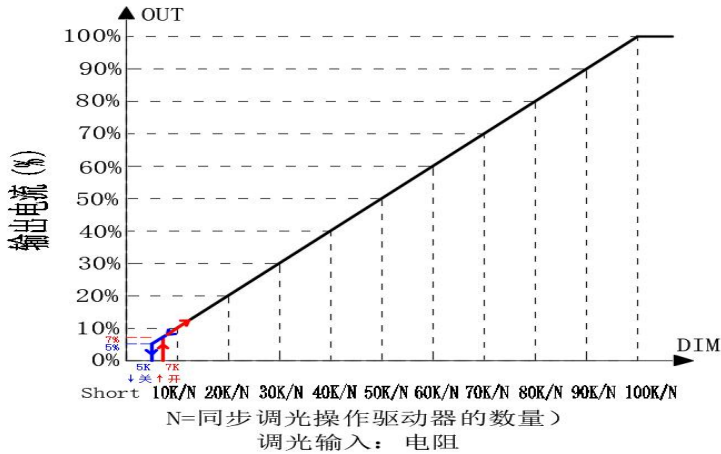
电阻调光（100K）
