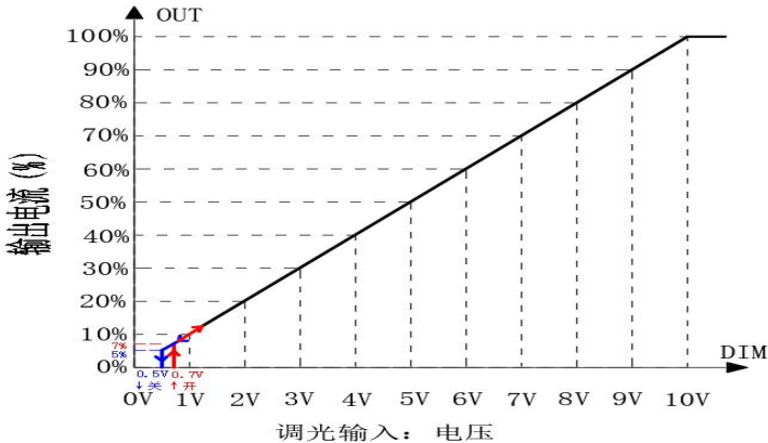
PWM调光（PWM频率 10V 1KHZ）
