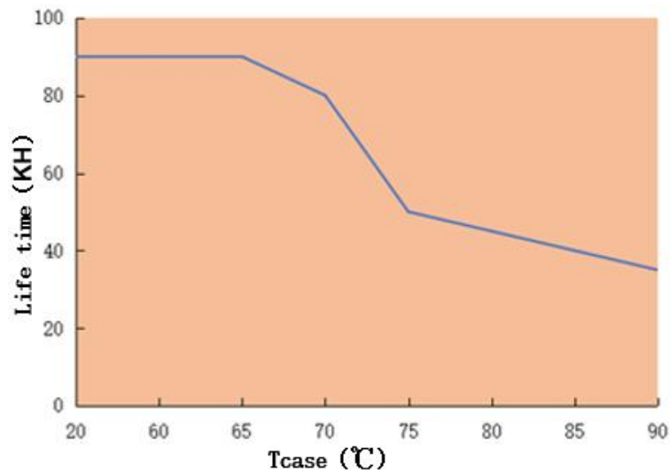
Tcase VS Life time LAG-200H-470A
