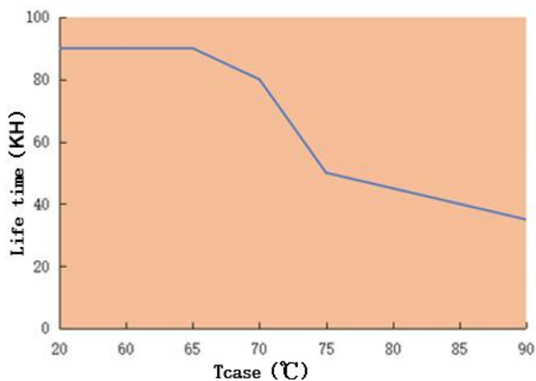
Tcase VS Life time LAG-80H-470A
