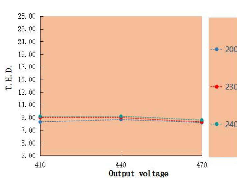
T.H.D. VS Output voltage LAG-80H-470A
