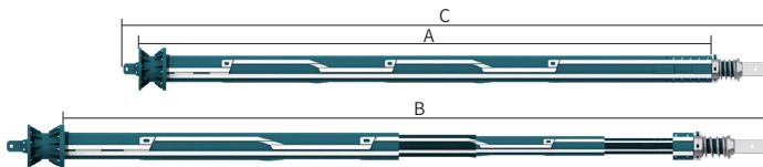
530系列钻杆型谱表 530 Series Kelly Bar Model List
