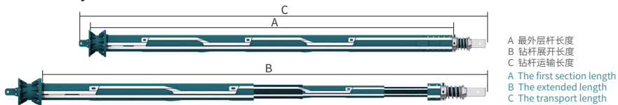
508系列钻杆型谱表 508 Series Kelly Bar Model List
