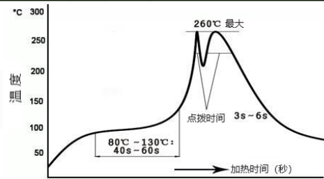
波峰焊曲线图
