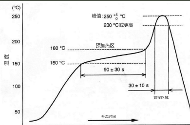
回流焊曲线图
