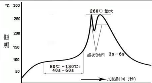
波峰焊曲线图
