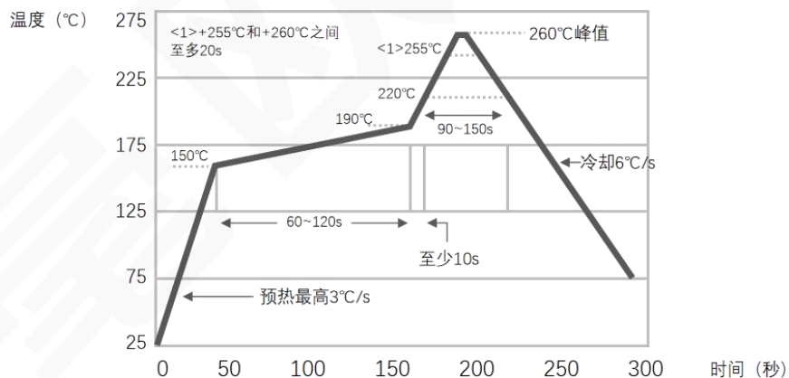
回流焊温度曲线
