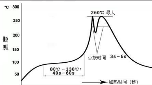
波峰焊曲线图
