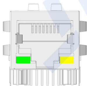
正视图 Front view
