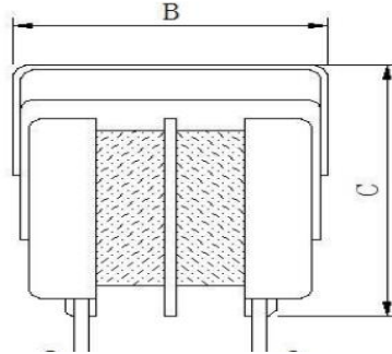
侧视图
