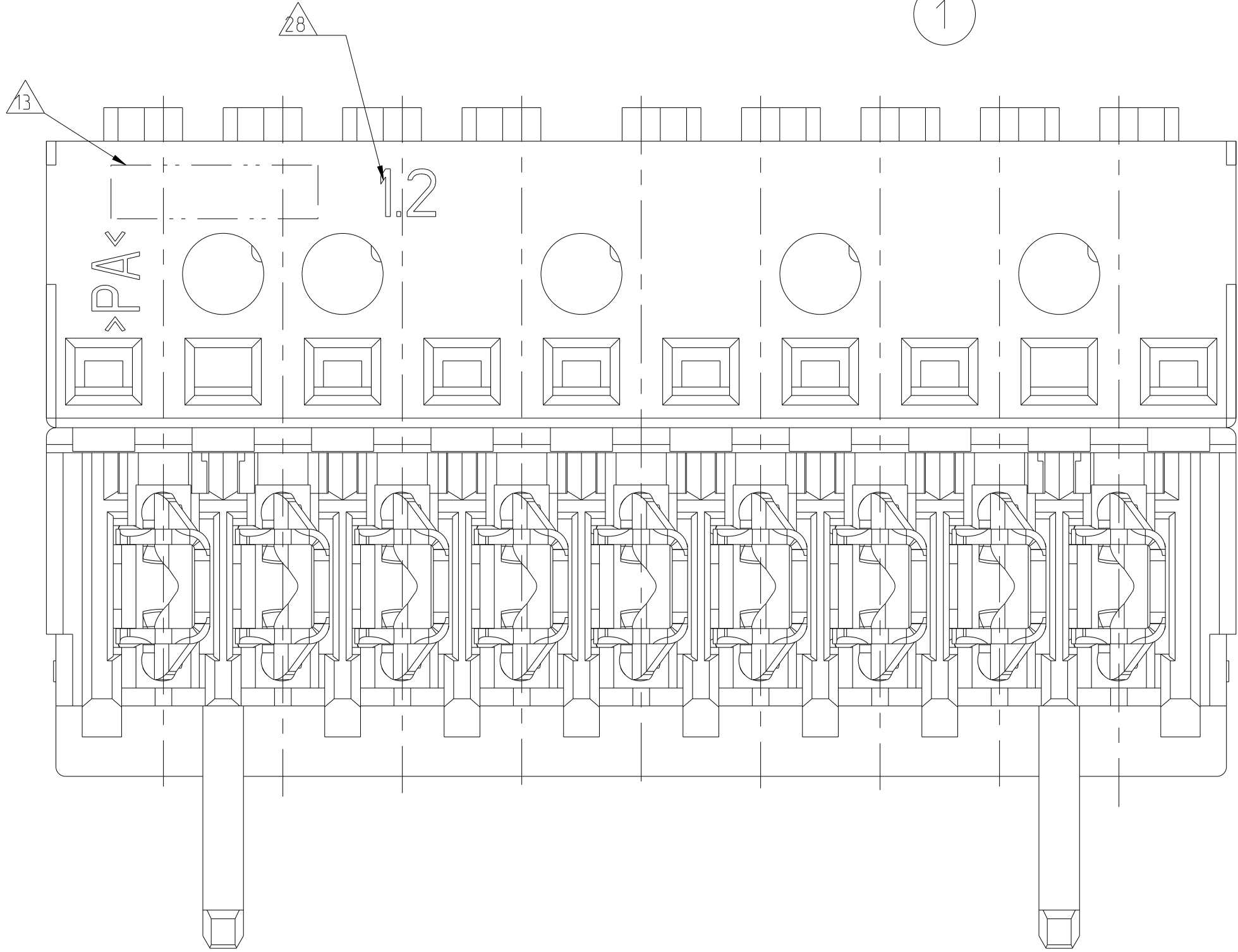
SECTION A-A
