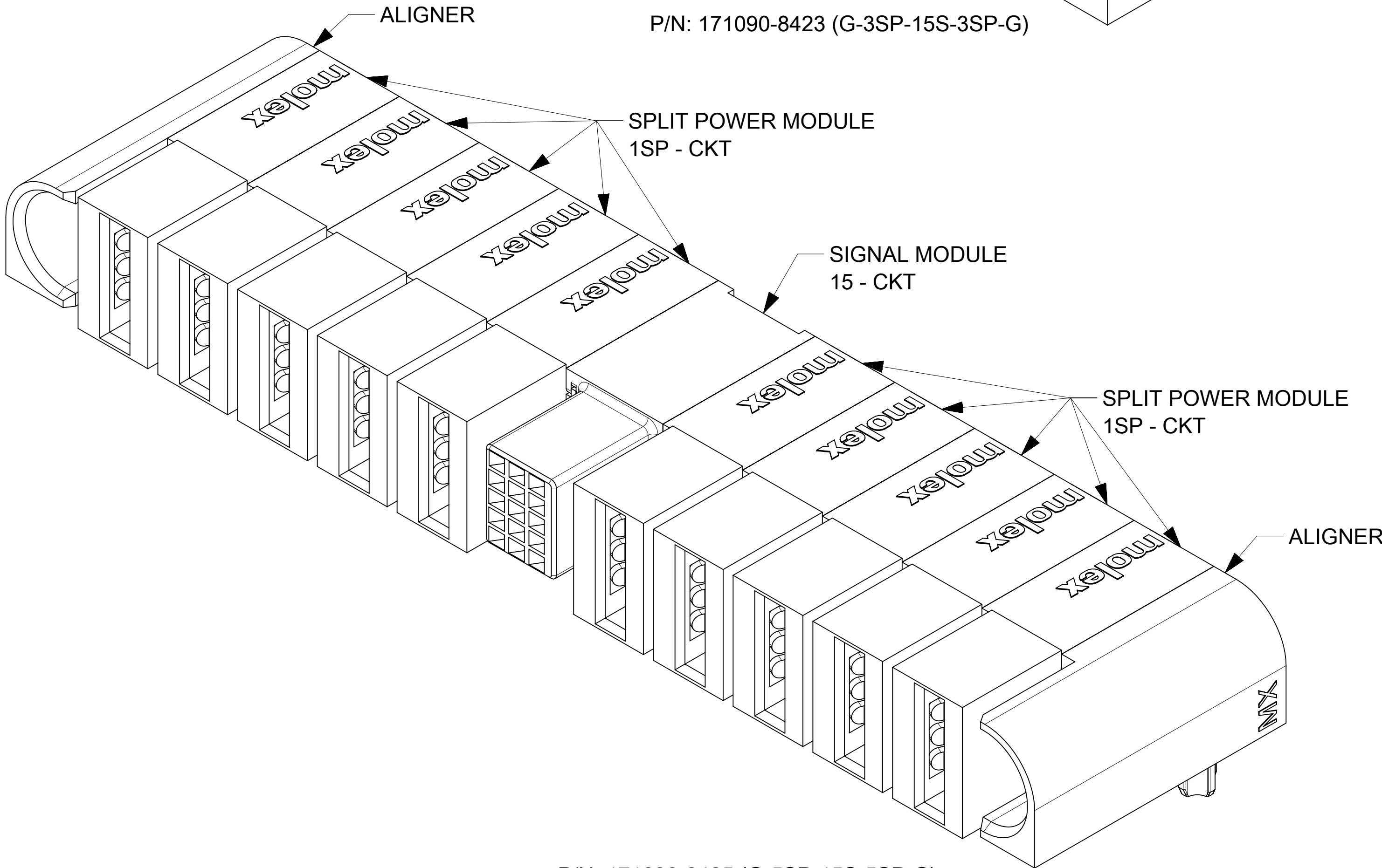
P/N: 171090-8425 (G-5SP-15S-5SP-G)
