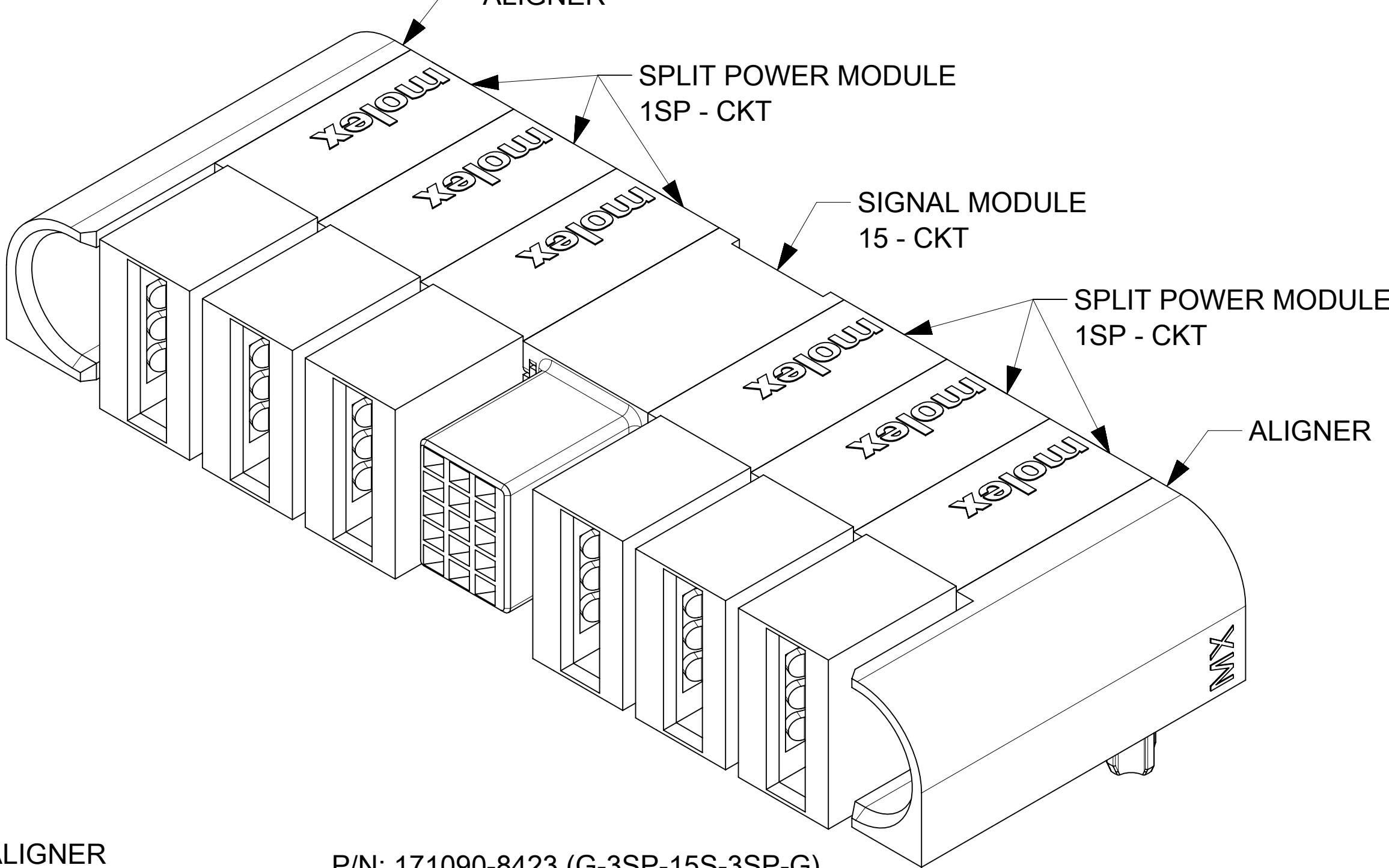
P/N: 171090-8423 (G-3SP-15S-3SP-G)
