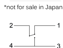
NC/NO function
