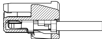
ターミナル装着図 TERMINAL ASSEMBLY DRAWING
