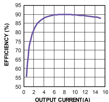
V_{IN}=12V, V_{OUT}=1.2V
