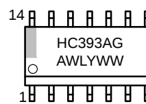
SOIC-14 NB
