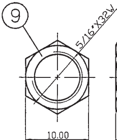
NUT
